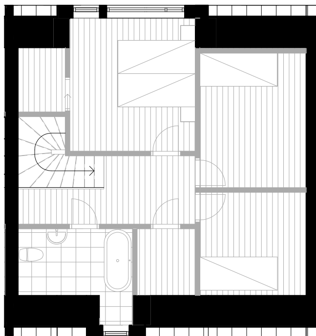
Plan 2tr, Möjlig vindsvåning
