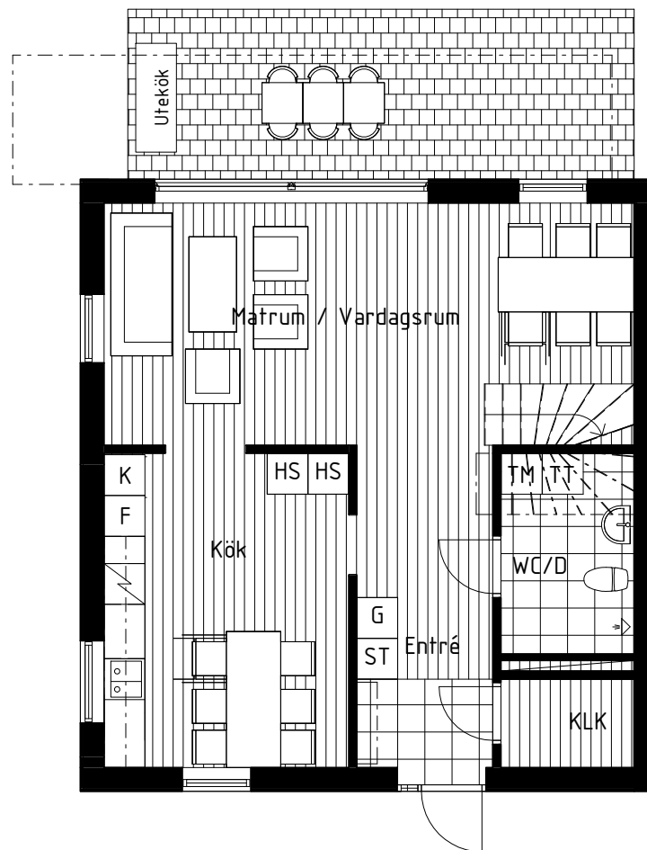
Plan 0, Entréplan
