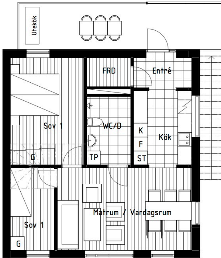
Plan 1tr, Entréplan
