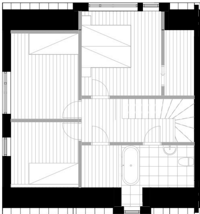
Plan 1tr, Entréplan
