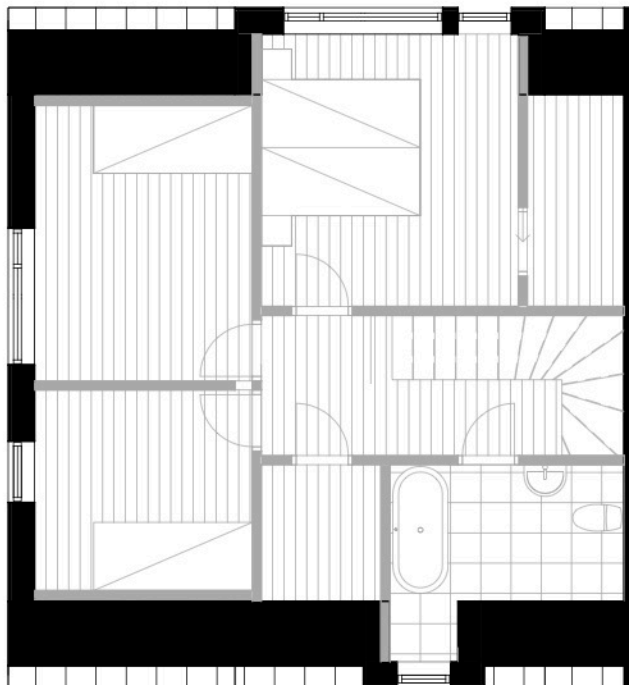
Plan 2tr, Möjlig vindsväning
