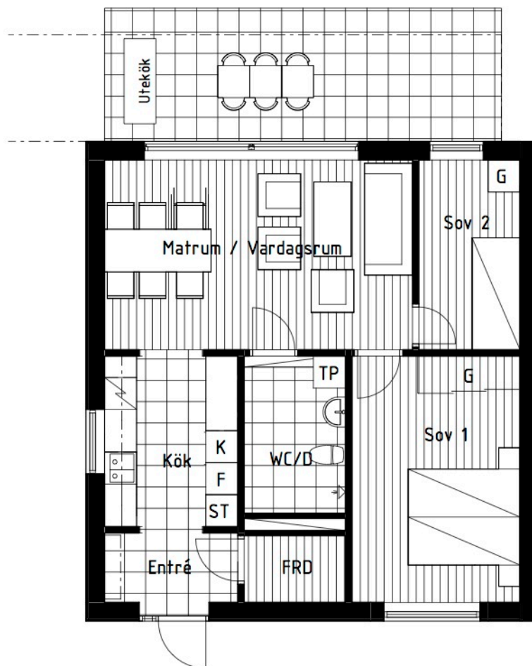
Plan 0, Entréplan
