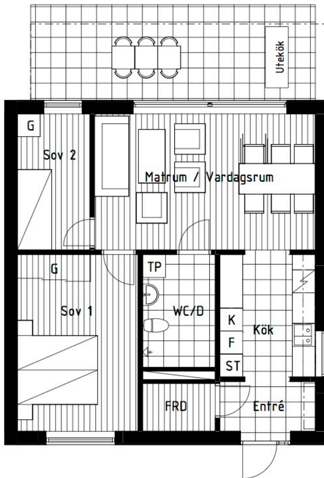
Plan 0, Entréplan
